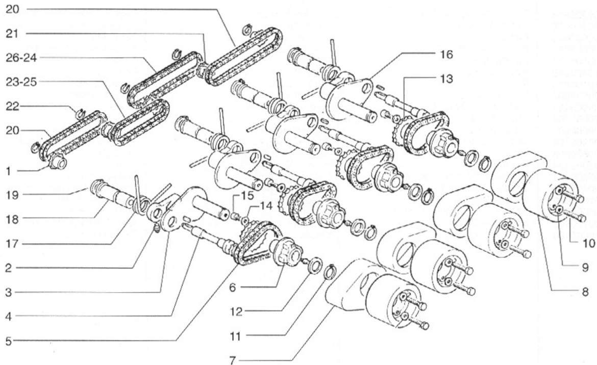
ABB. 2 - ÜBERTRAGUNGSEINHEIT TAB. 2 - TRANSMISSION GROUP PL. 2 - ENSEMBLE TRANSMISSION
