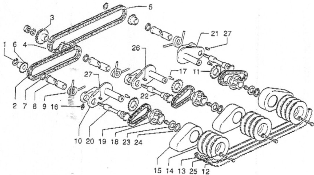
ABB. 4- ÜBERTRAGUNGSEINHEIT TAB. 4- TRANSMISSION GROUP PL. 4- ENSEMBLE TRANSMISSION (VS 34 C1)
